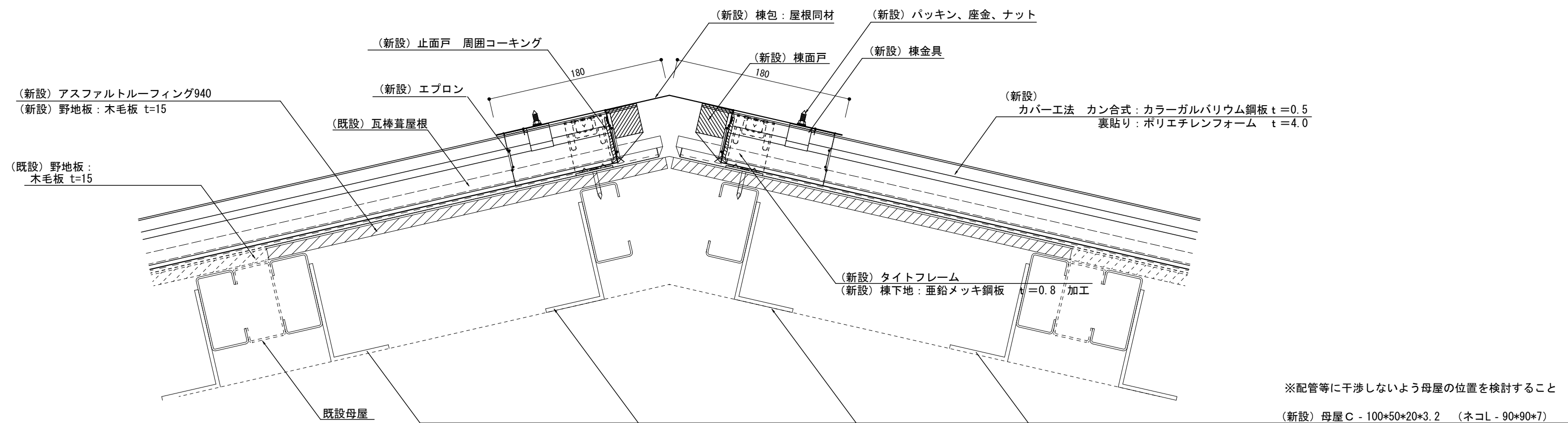
換気棟撤去後改修詳細図
