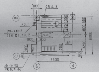
配置平面 S=1/100
