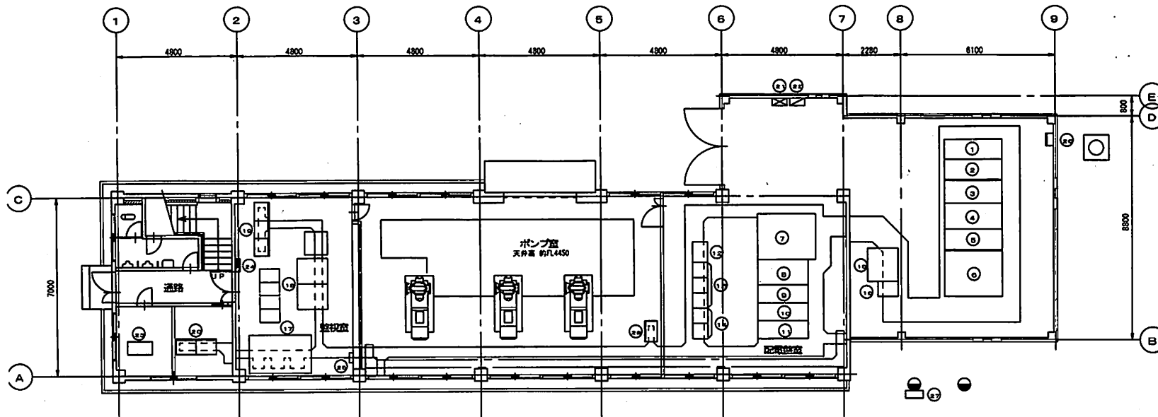
田口山配水場 1F 平面図
