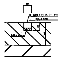
止水溝詳細図 S=1/10
