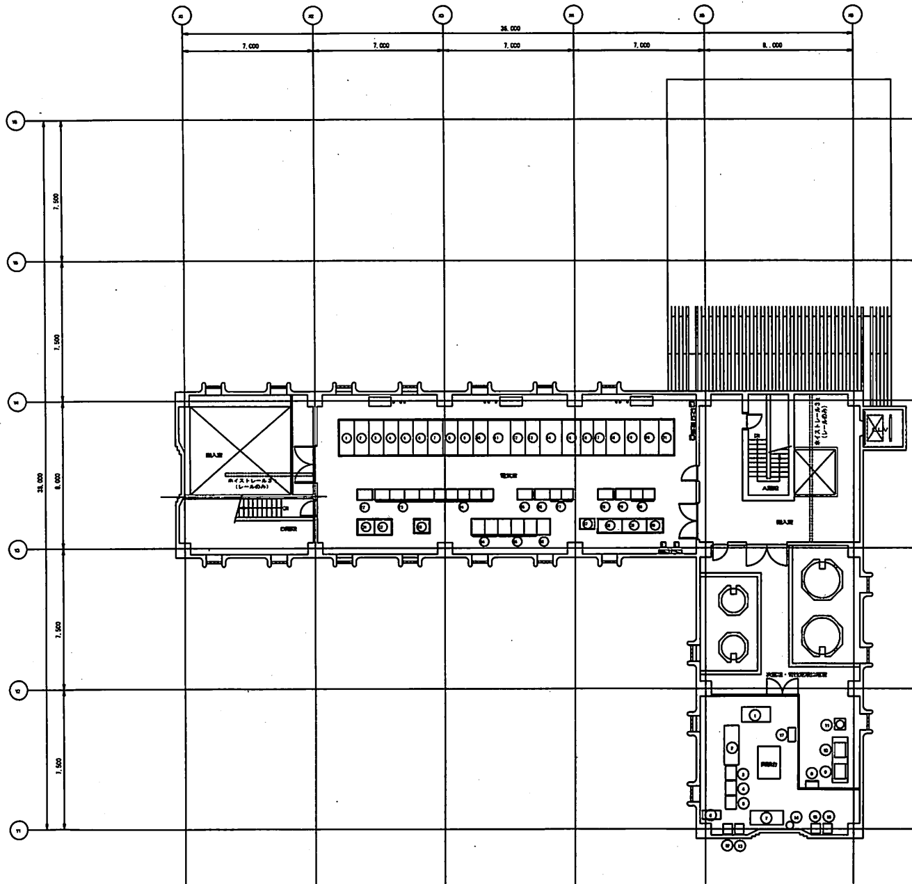
2 階 平 面 図
