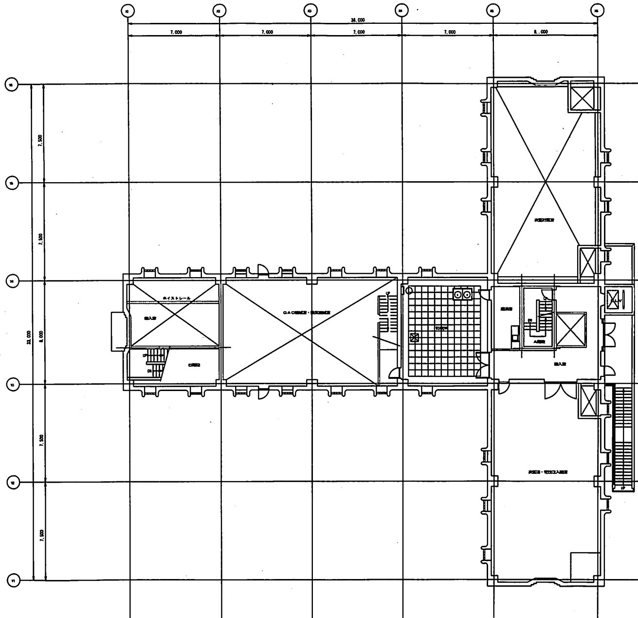
1 階 平 面 図
