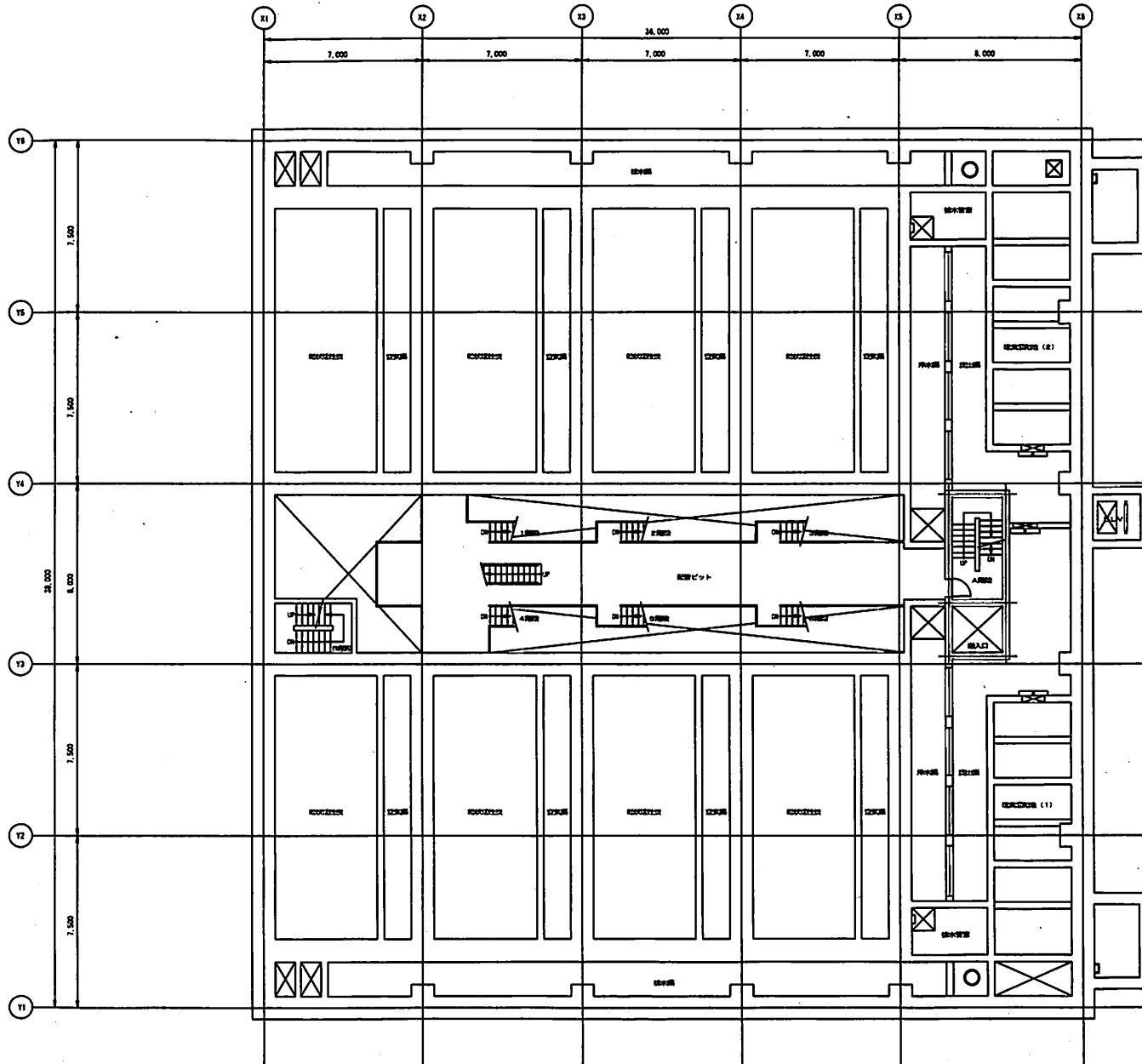
地下1層 下部
