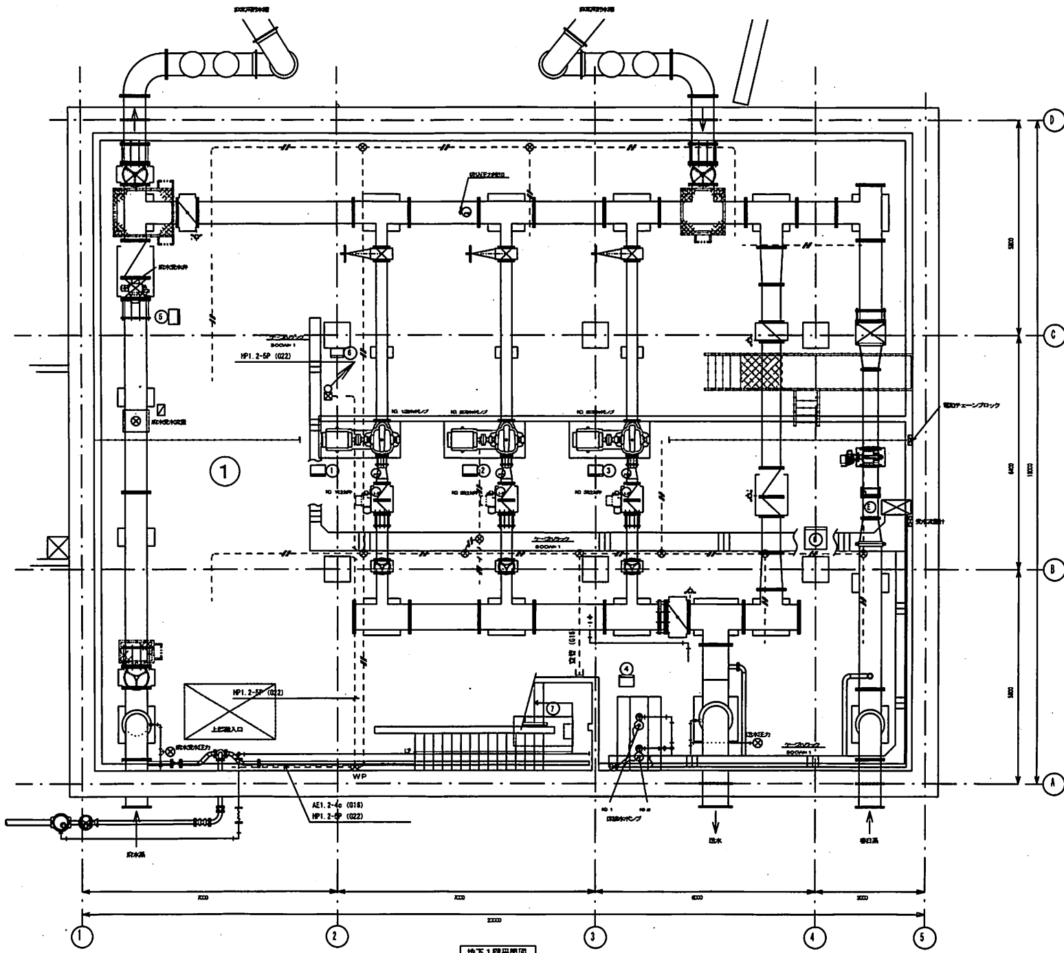
地下1階平面図 天井高6m
