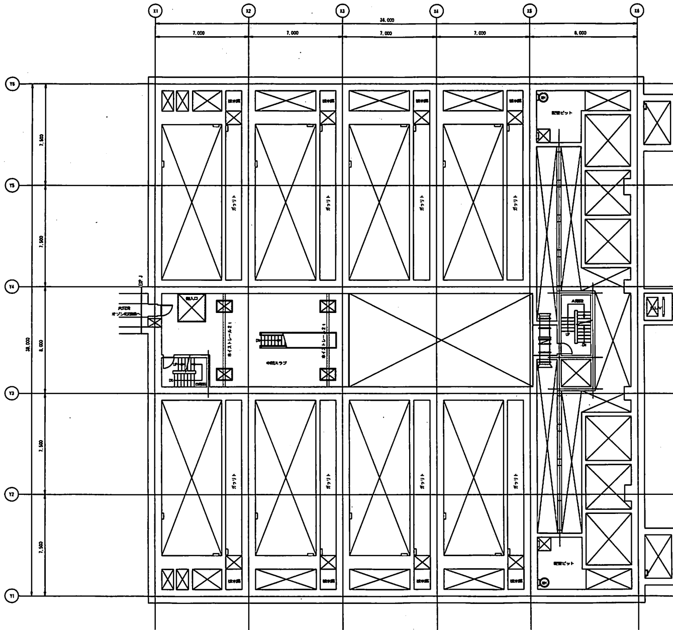
地下1層 上部
