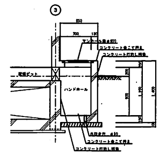
ハンドレール詳細図 S=1/30
