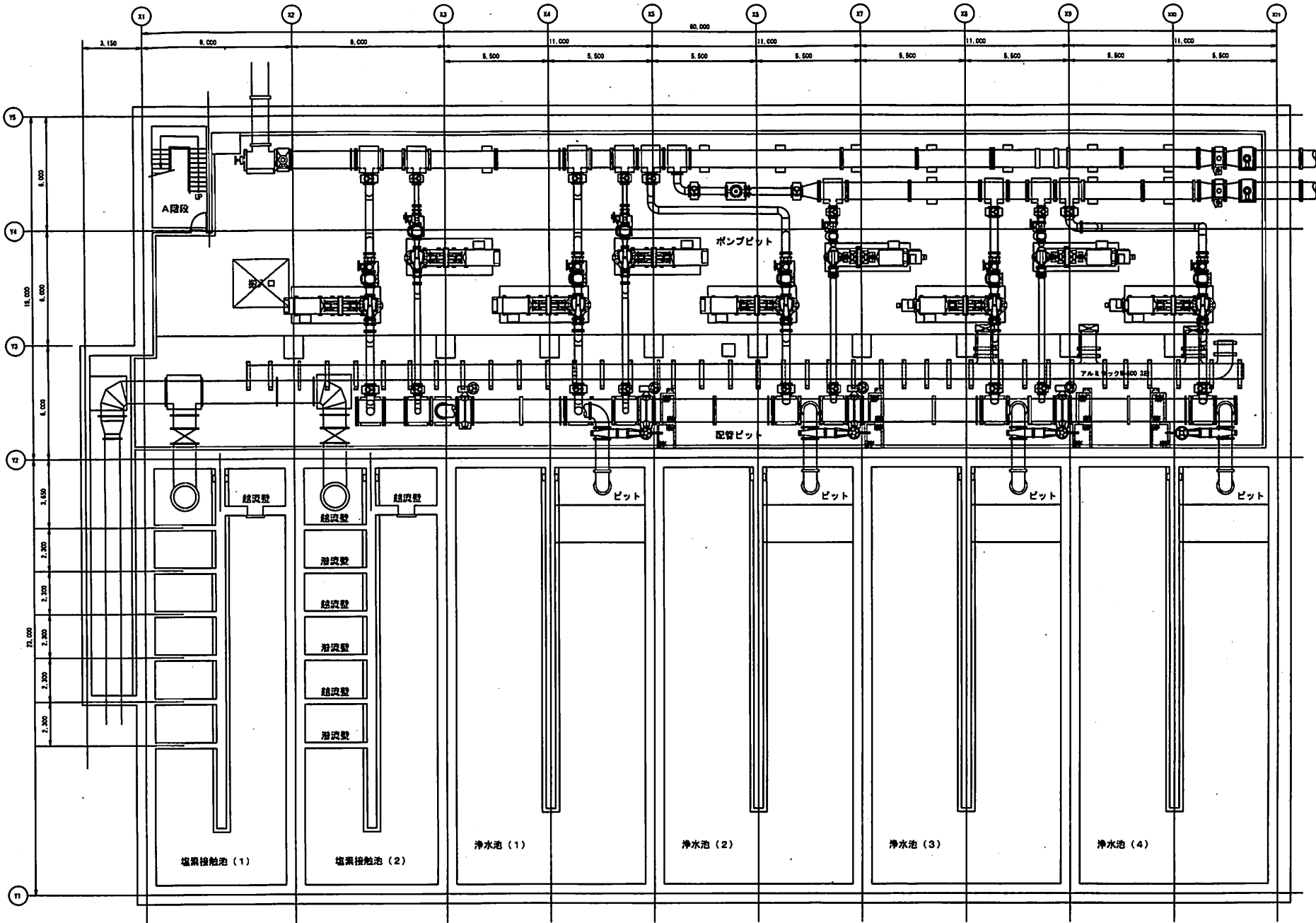
地下2層 平面図
