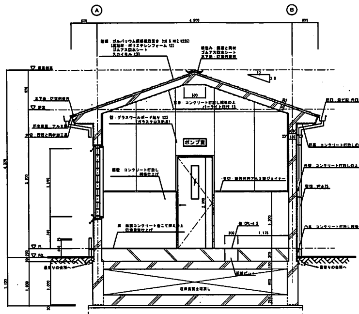
理計図 S=1/30
