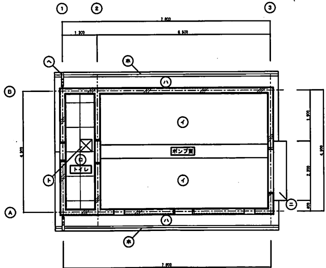
天井伏図 S=1/50
