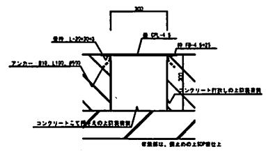
配線ピット詳細図 S=1/10
