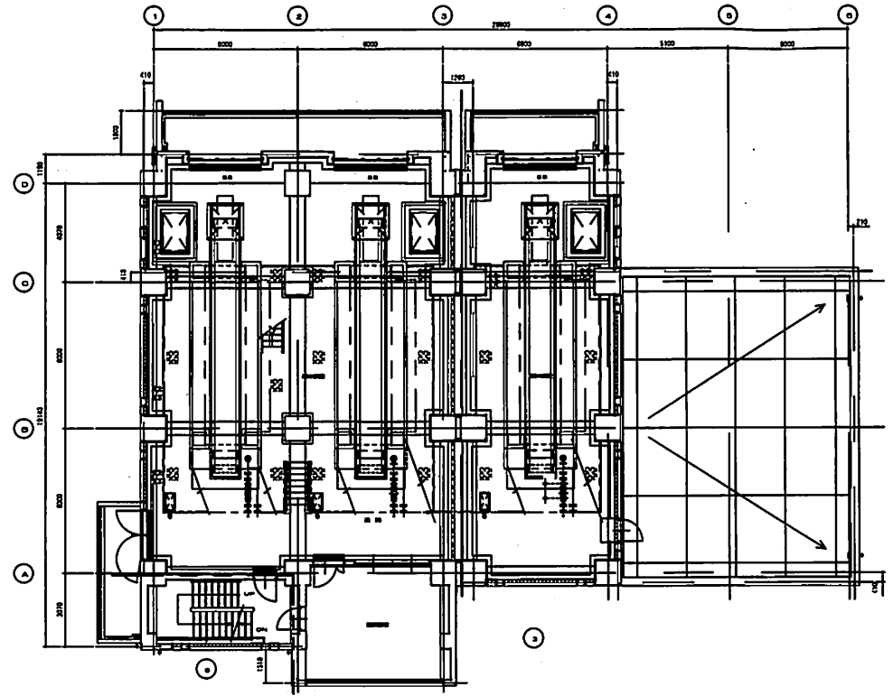
1階・2階 縮尺=1/200
