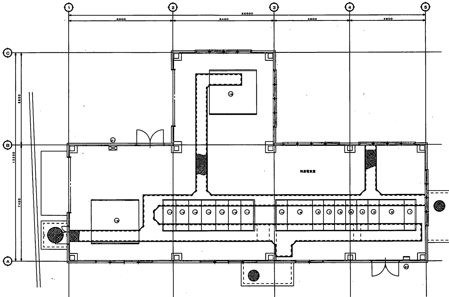
特高電氣室平面図 S:1/100
