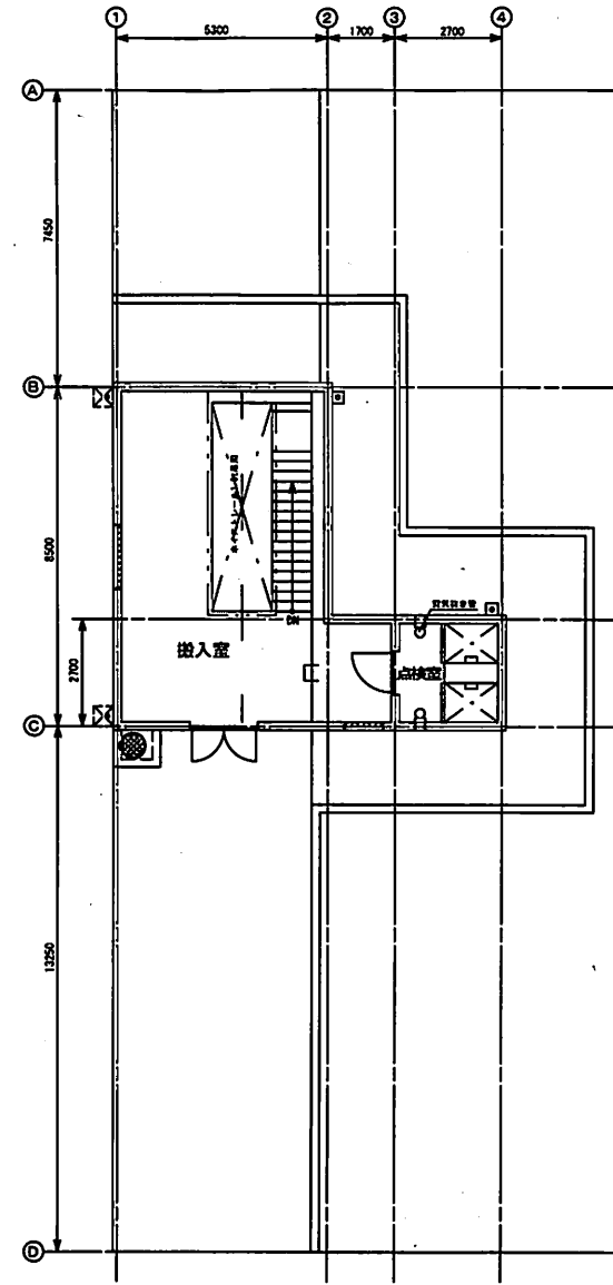
1階 平面図
