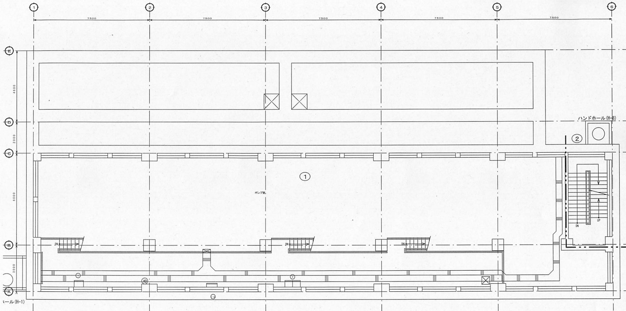
ポンプ室平面図 S:1/100
