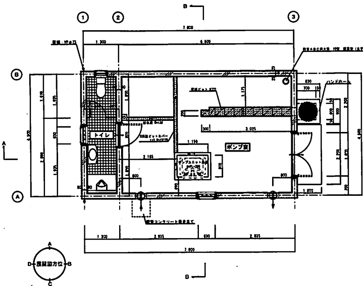
平面詳細図 S=1/50
