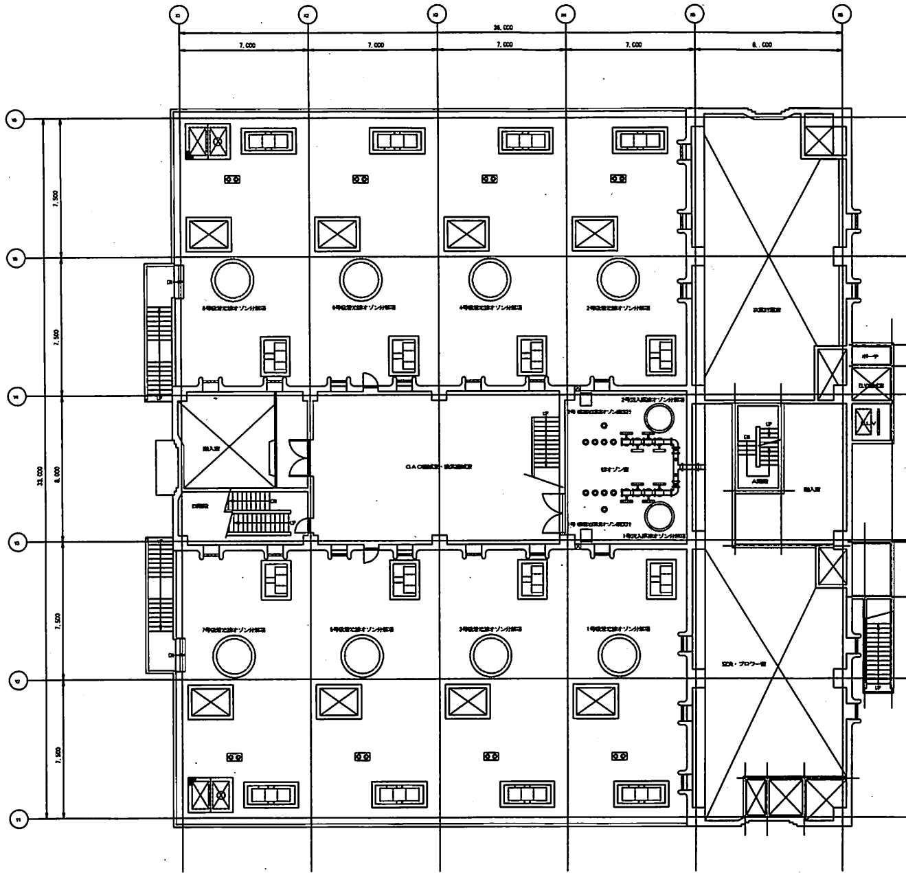
L1階平面図
