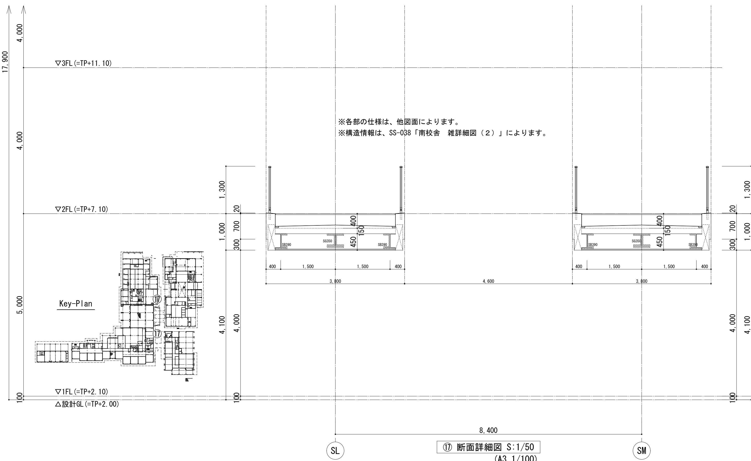
別図2 「屋外渡り廊下 断面図」
