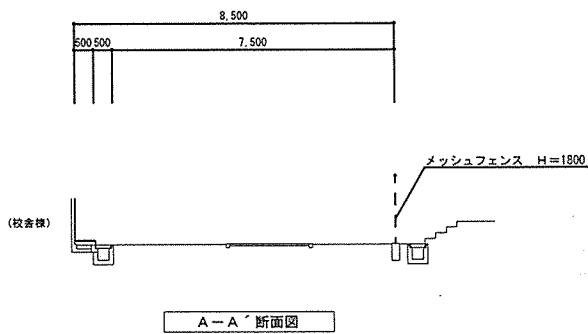
A-A' 断面図
