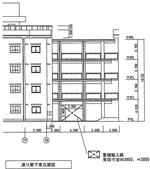
渡り廊下東立面図
