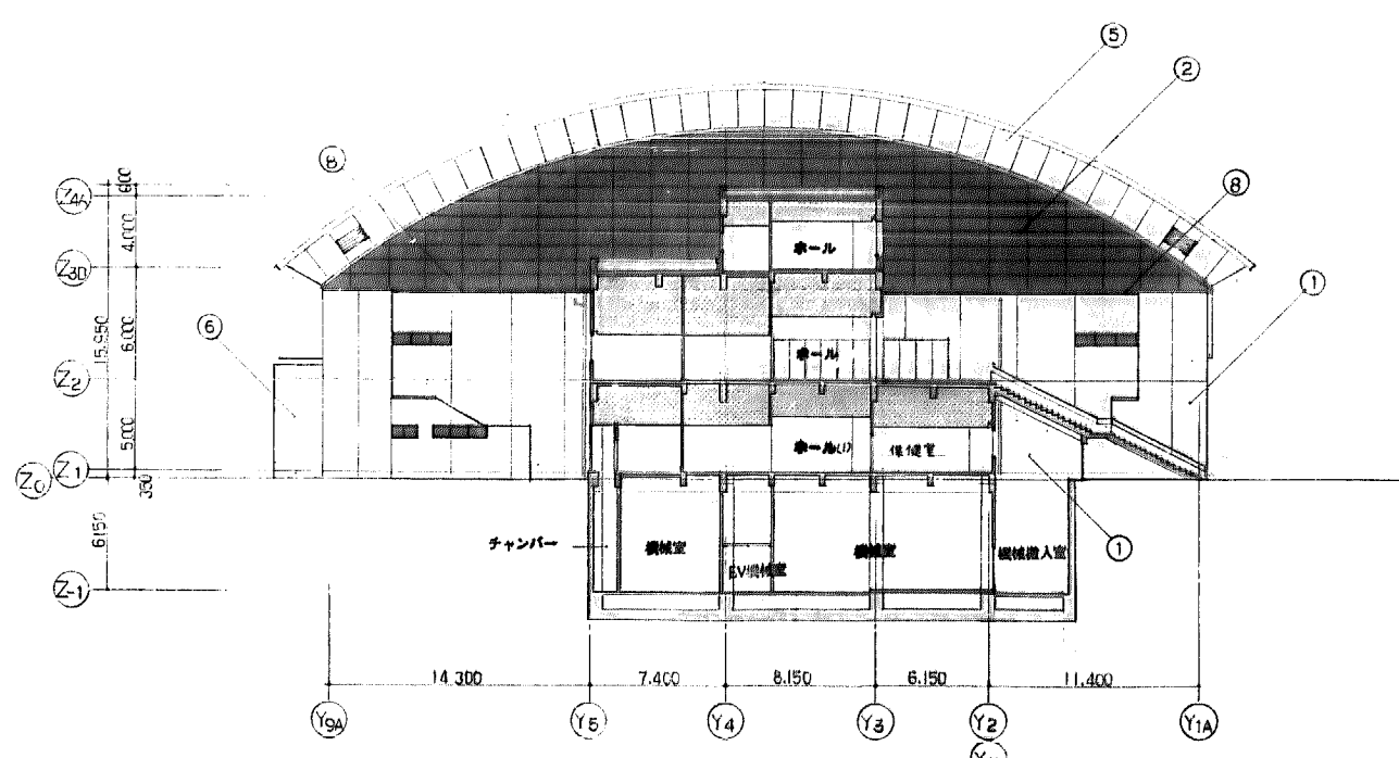
断面図 1:200
