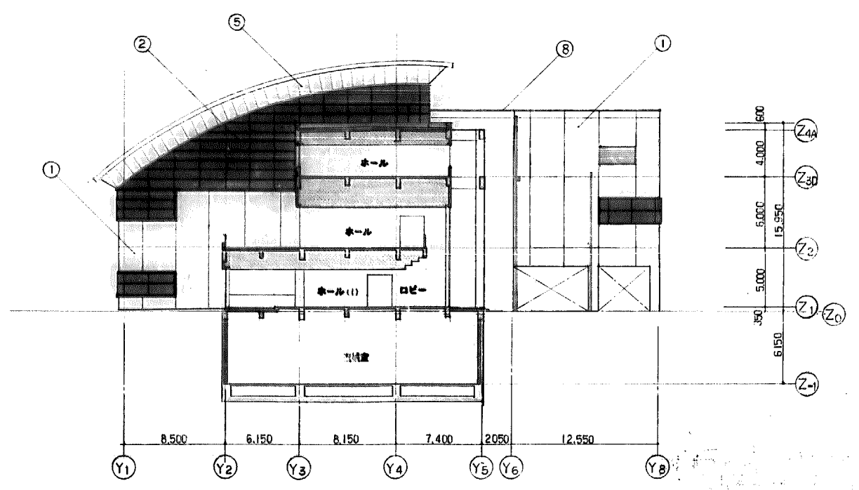
断面図 1:200
