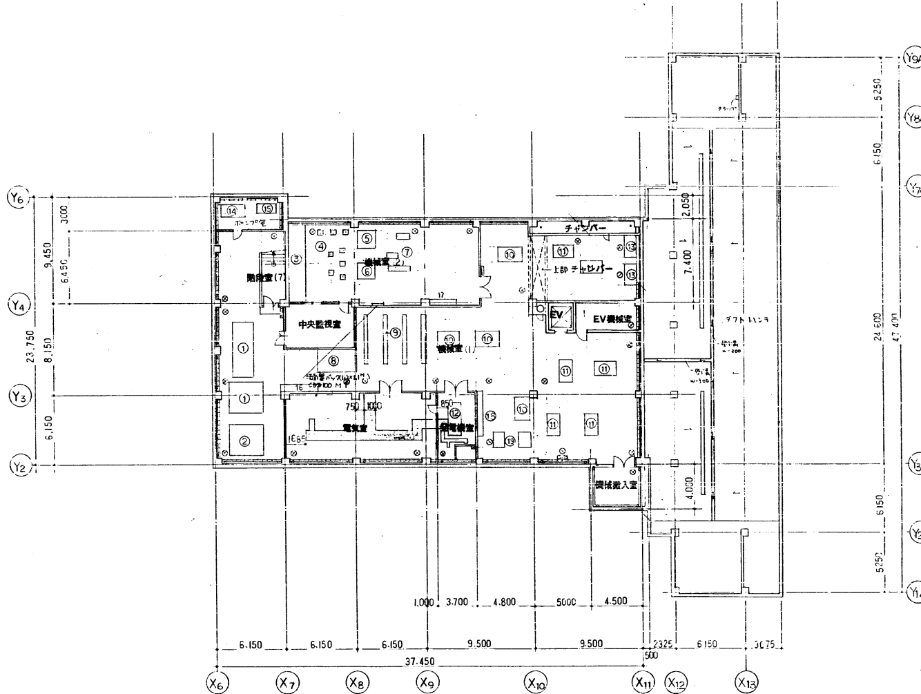
B1階平面図 1:200
