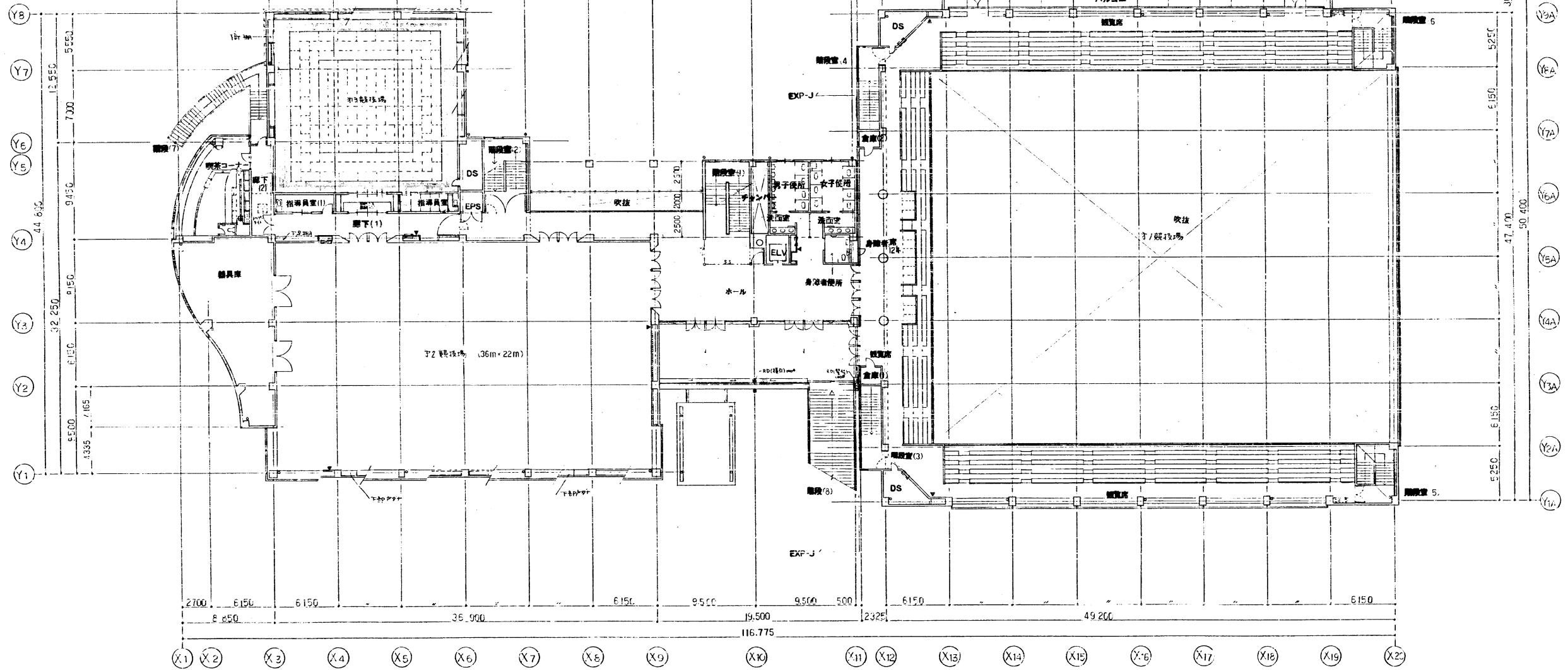
2階平面図 1:200
