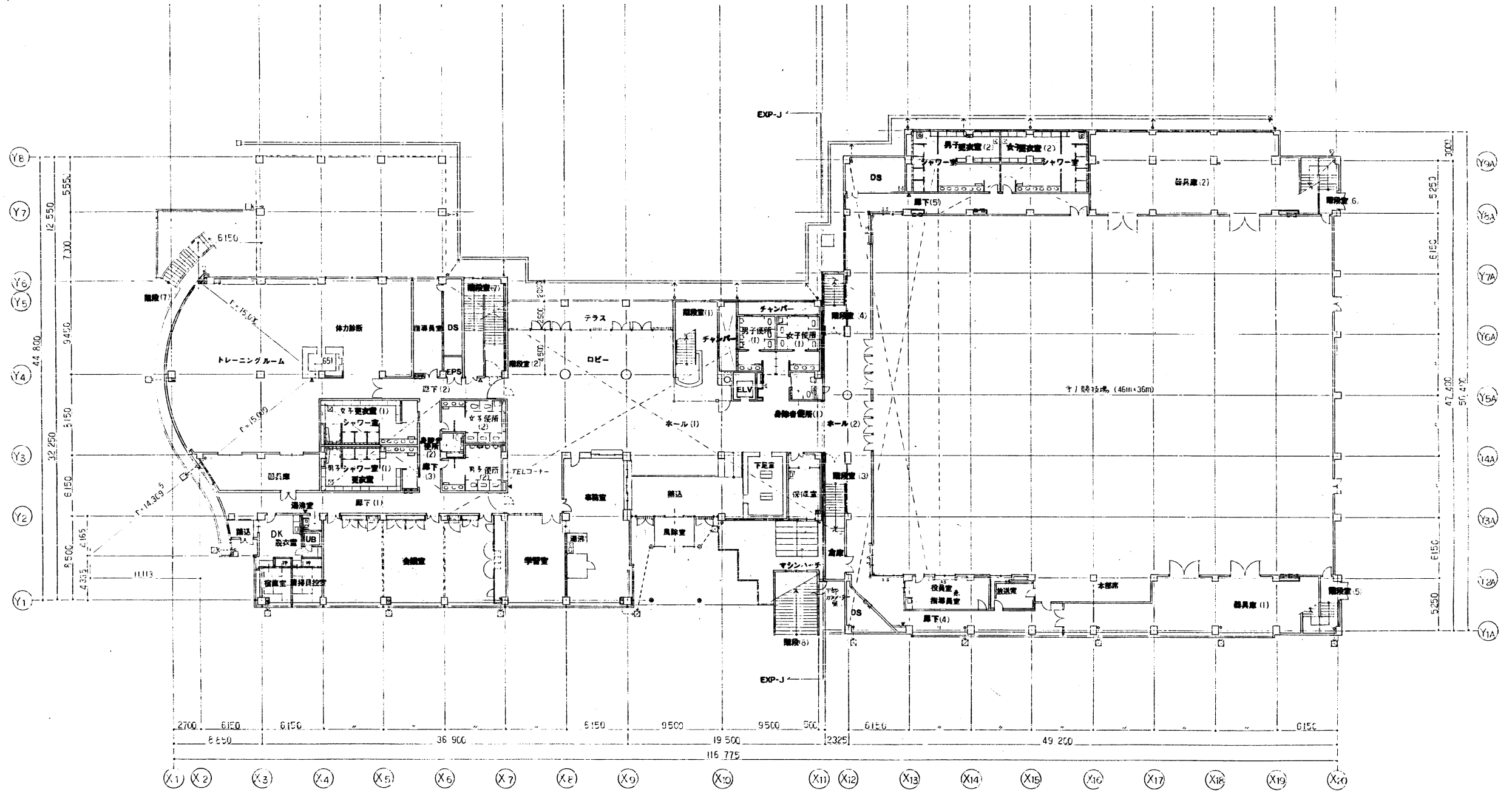
1階平面図 1:200
