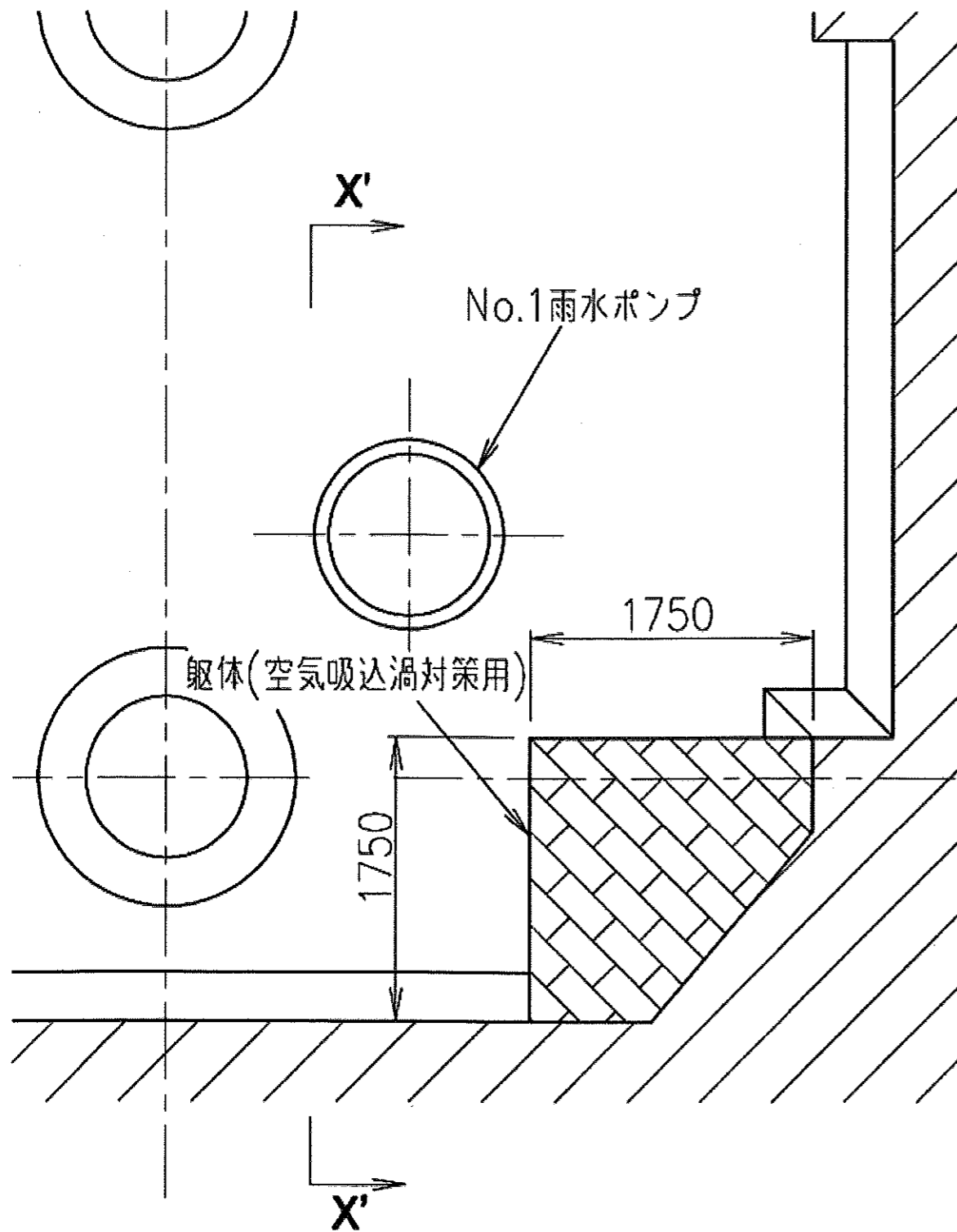
図 15 渦流防止対策 (空気吸込渦対策用)
