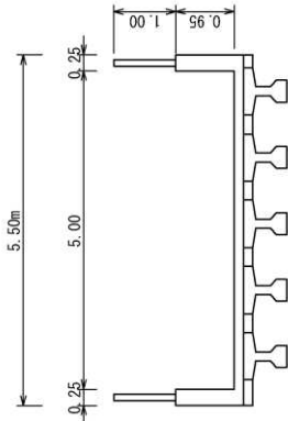
第3, 4径間
