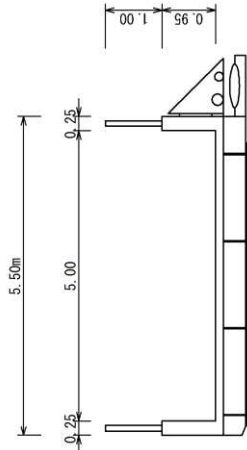
第2径間
