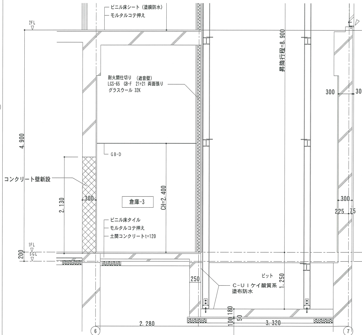
EVピット矩計図 S=1/30
