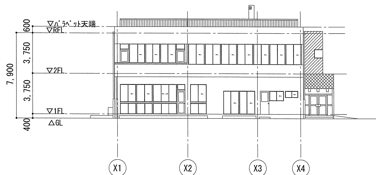
改修後 南立面図 1:200
