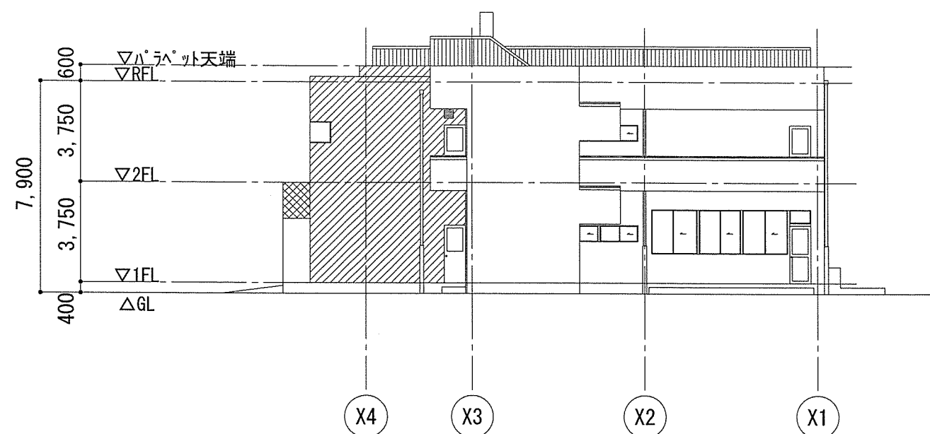
改修後 北立面図 1:200
