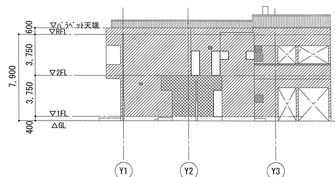
改修後 東立面図 1:200
