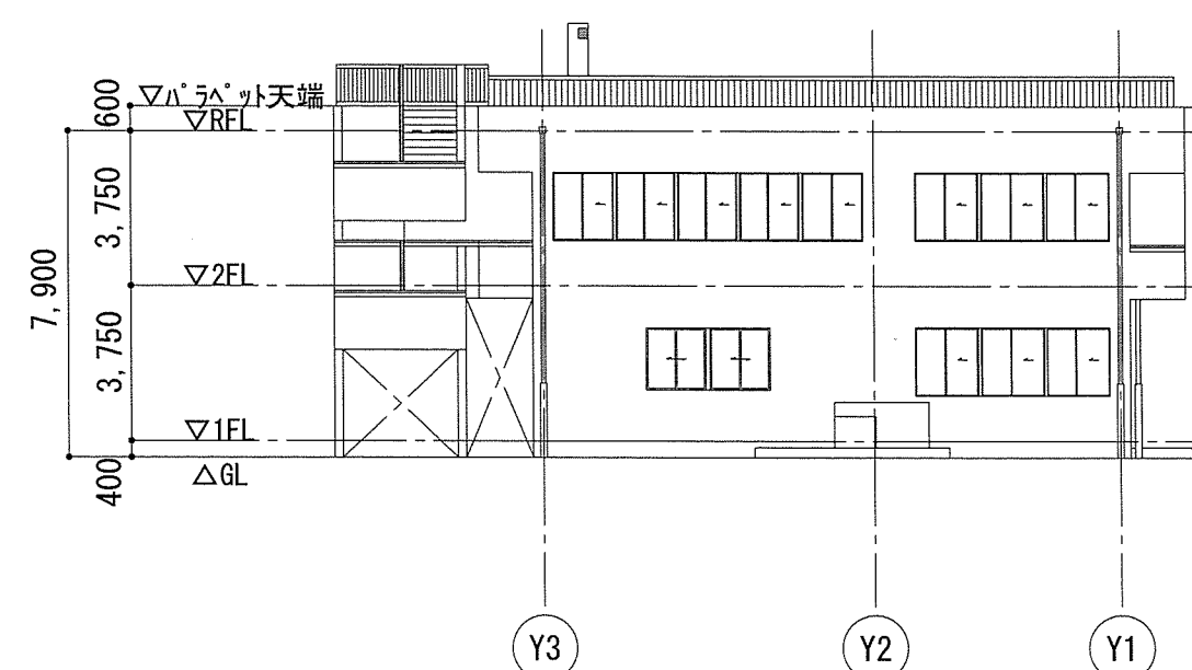
改修後 西立面図 1:200
