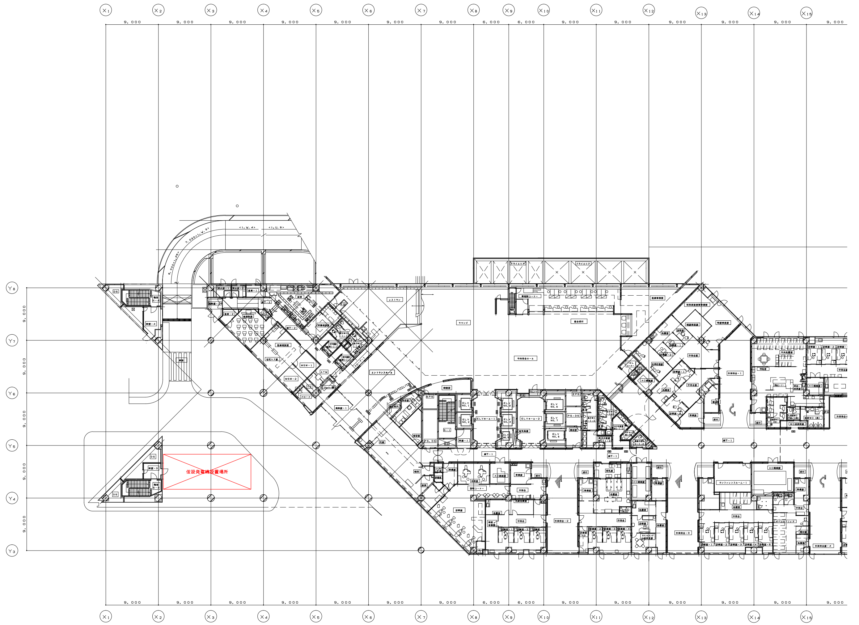
1 階平面図
