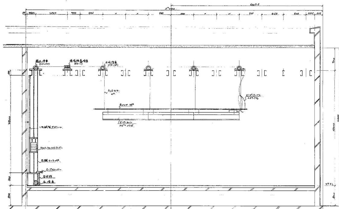
吊钩装置正面详图 Y30
